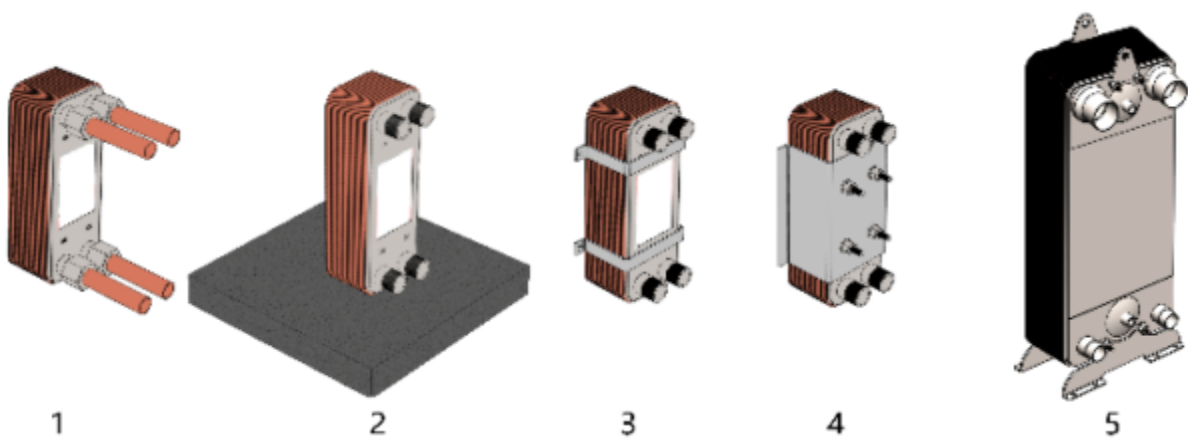
Рис.7 - Рекомендации по монтажу теплообменников ВРНЕ 1. Крепление непосредственно на трубопровод (маленькие модели); 2. Опора снизу; 3. Монтаж на кронштейн из листового металла (резиновая вставка между кронштейном и теплообменником); 4. Монтаж при помощи монтажных болтов на торцевой пластине; 5. Для больших теплообменников доступны опоры в комплекте.
